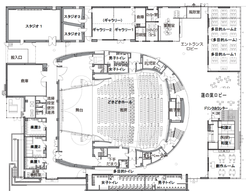
【1階平面図】
